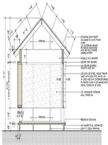
SECTION ELEVATION 'B-B'
